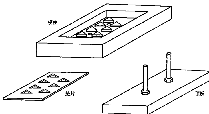
图6 灰锥托板模
