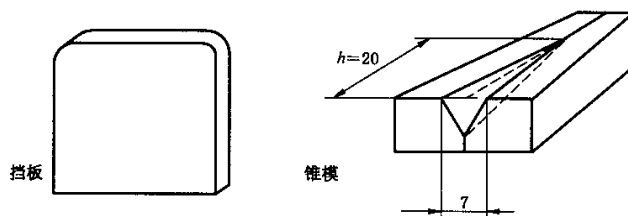
图5 灰锥模子
