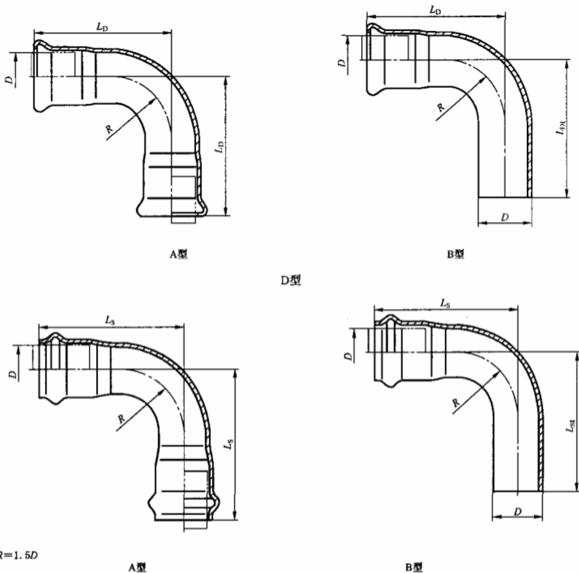
S型 图 7 90°弯头
