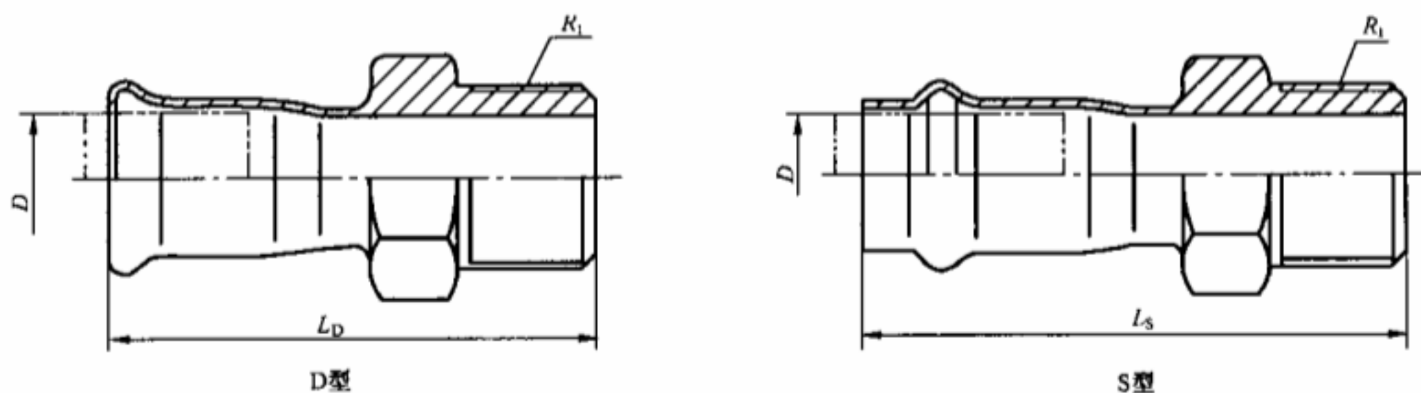
图10 外螺纹转换接头
