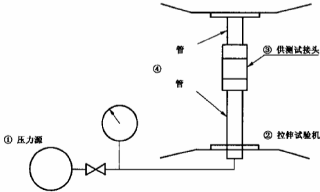
图 11 拉拔试验装置
