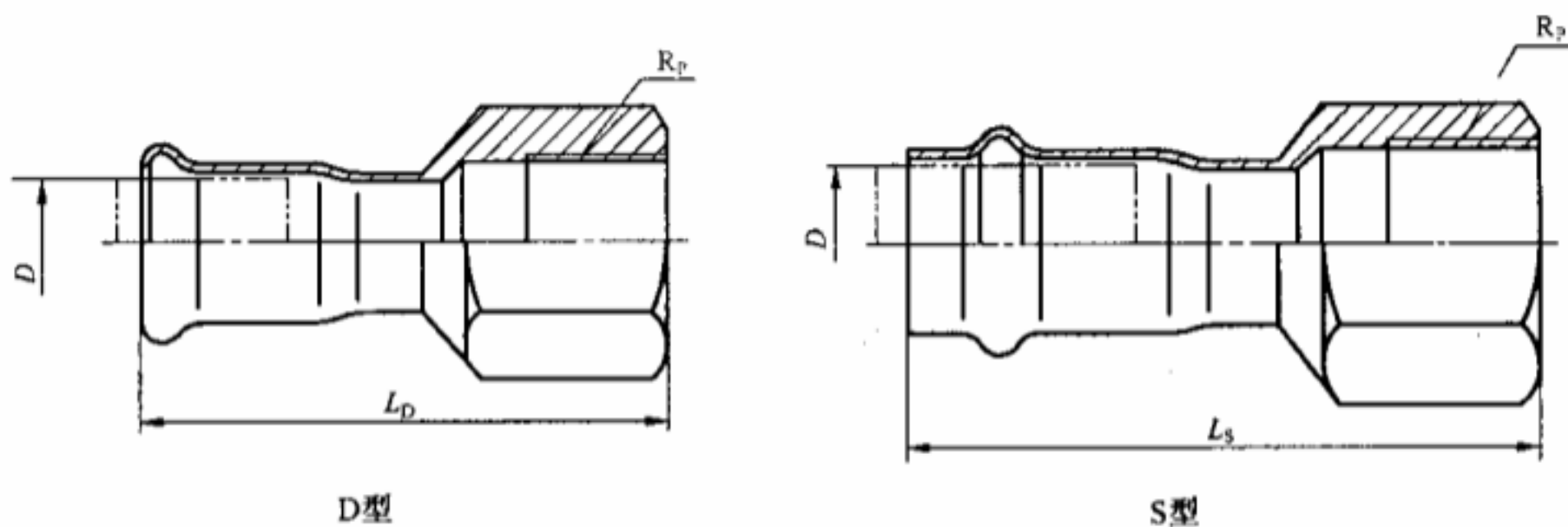
图 9 内螺纹转换接头
