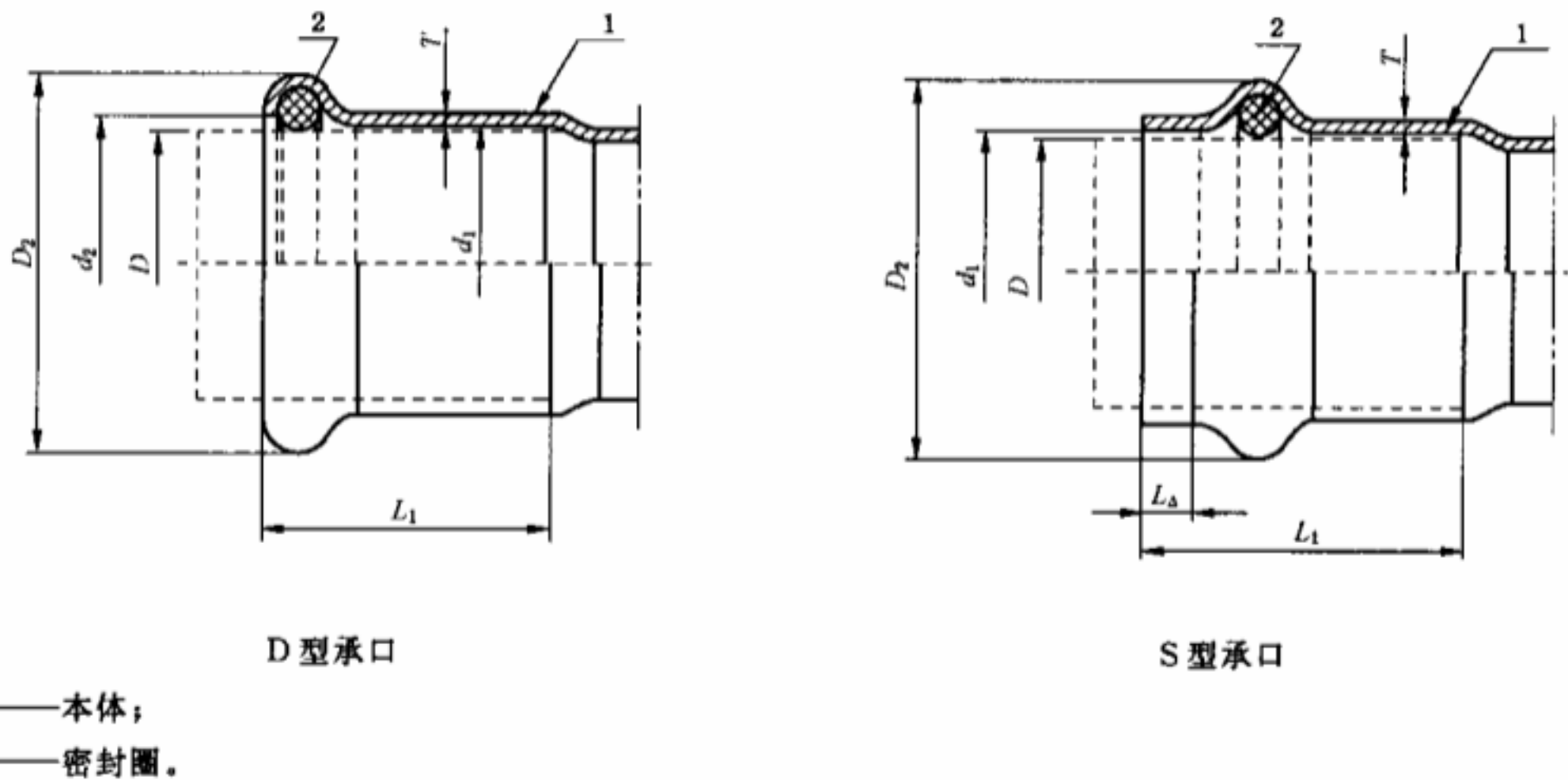
图 1 卡压式管件承口
