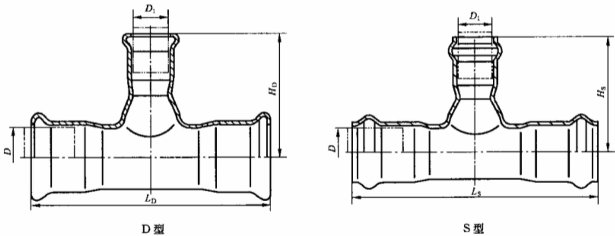
图 6 异径三通
