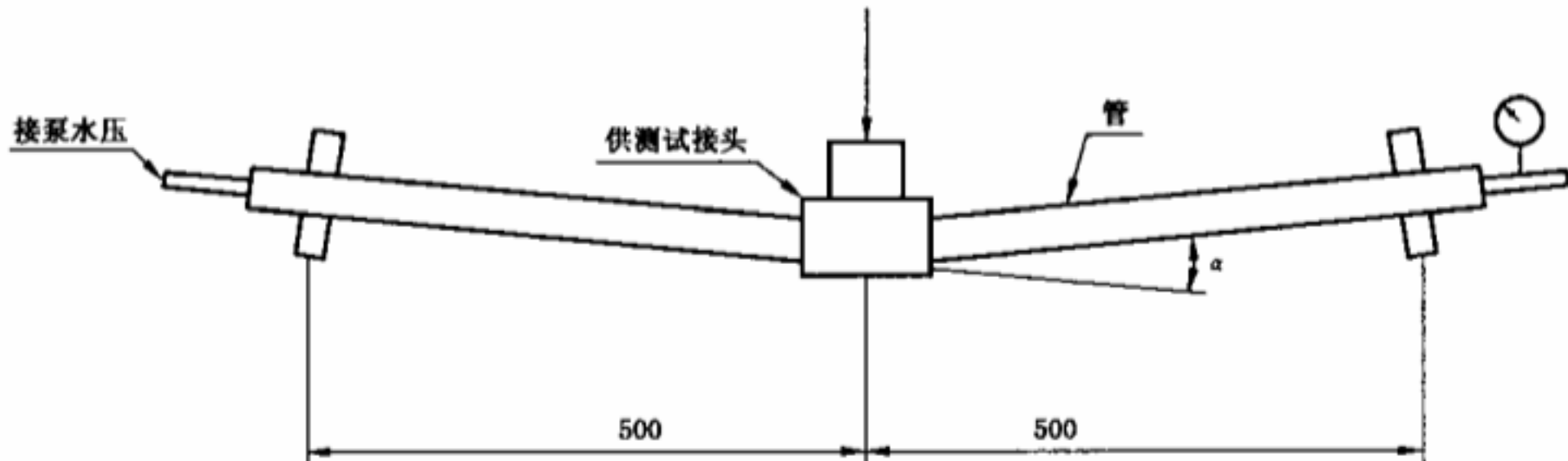
图 13 水压弯曲挠角试验装置
