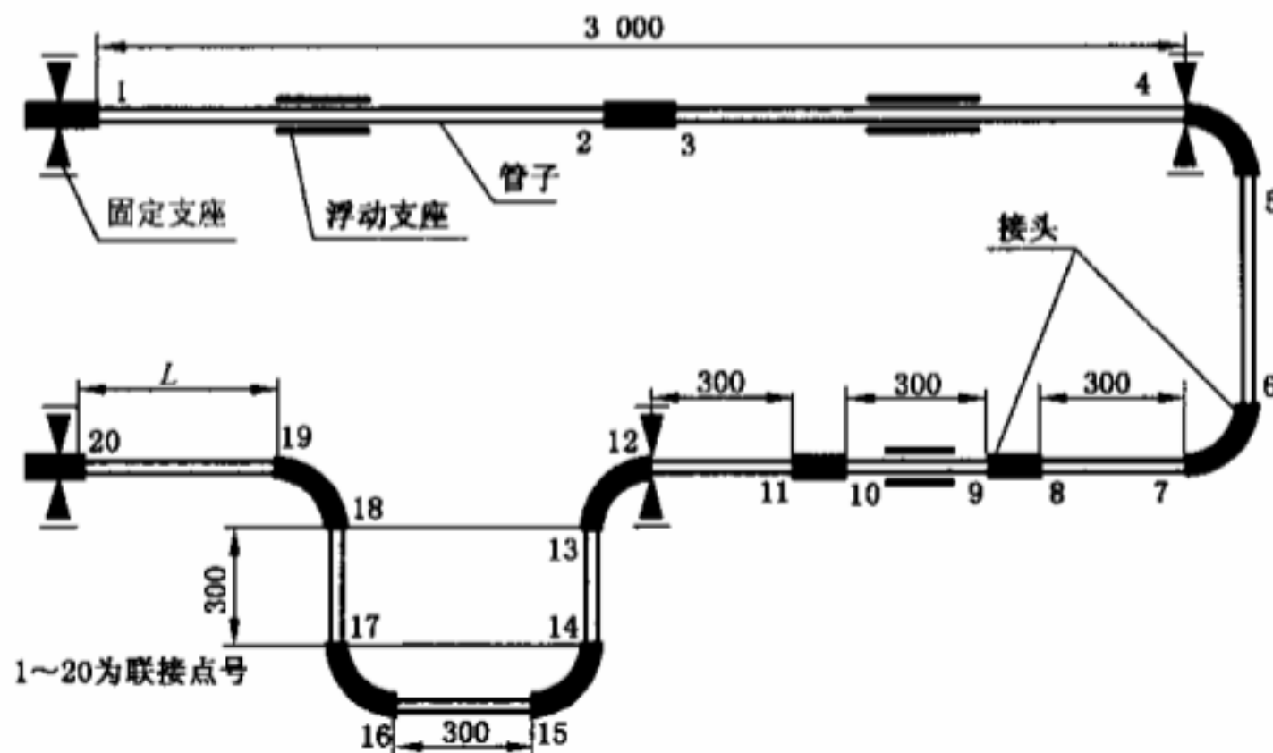
图 12 温度变化试验装置
