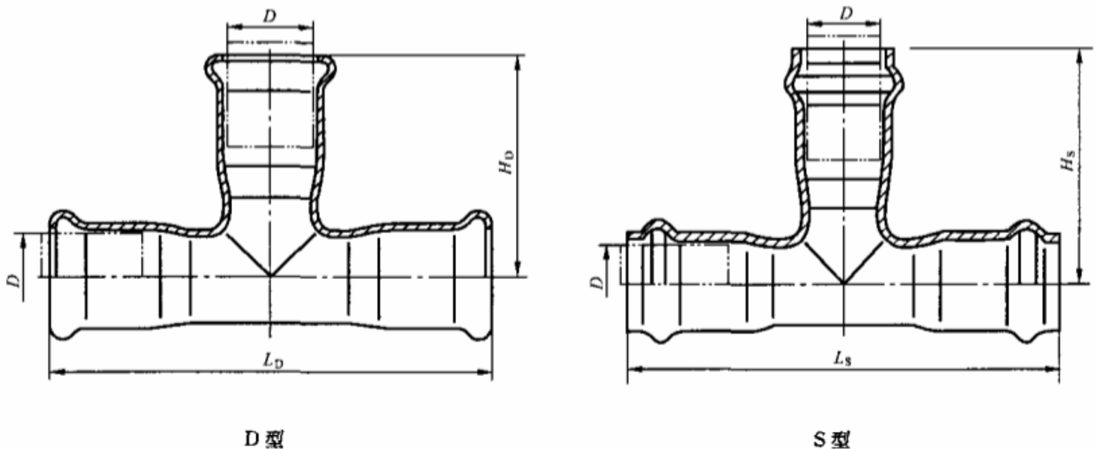
图 5 等径三通
