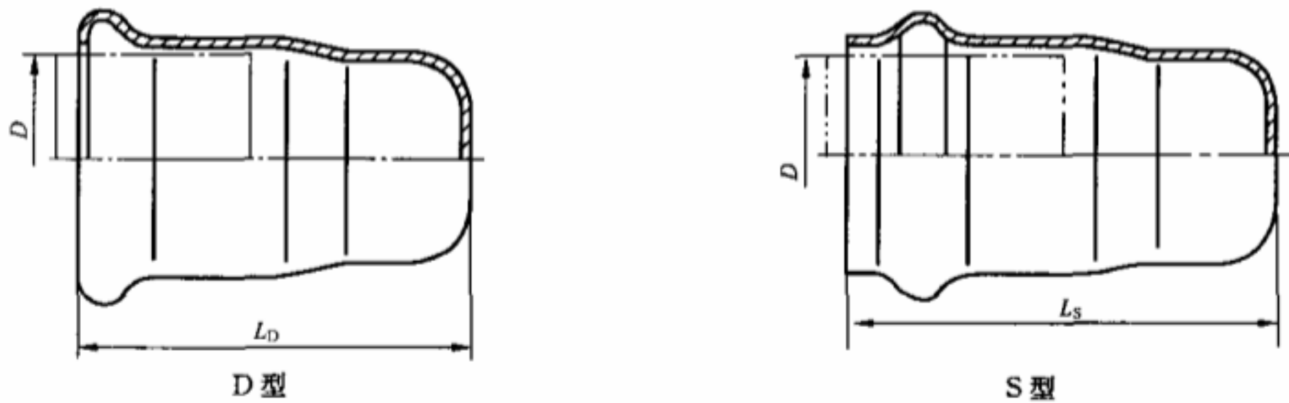
图2 管帽
