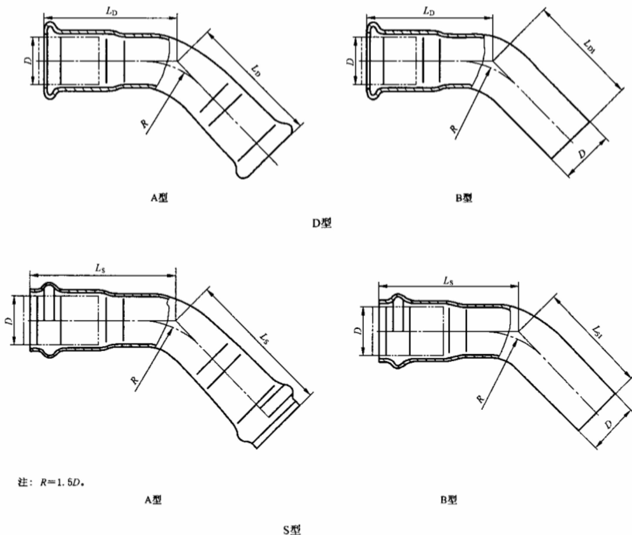
图 8 45°弯头
