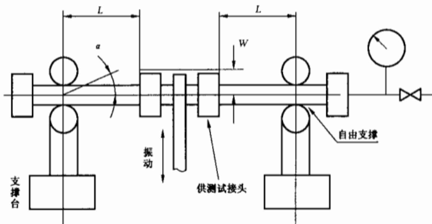
图 14 振动试验装置
