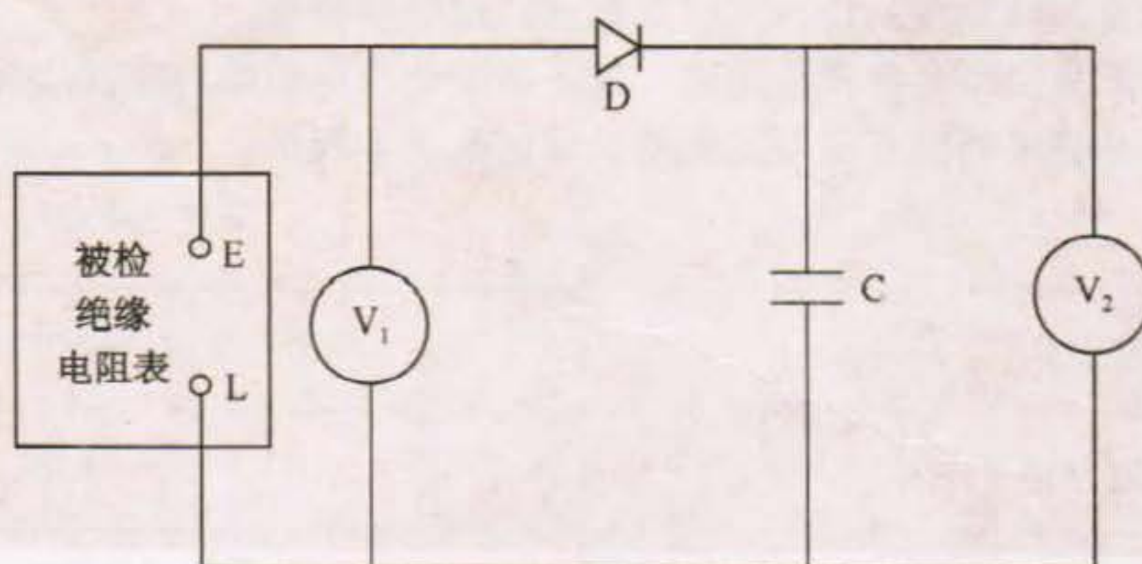
图2 绝缘电阻表基本误差检定接线图
